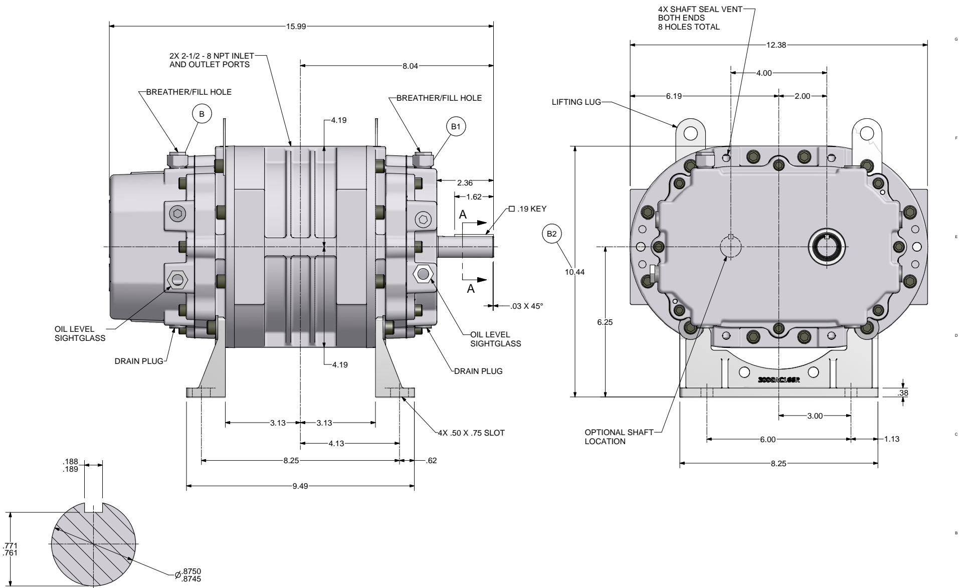
SECTION A-A SCALE 4 : 1
