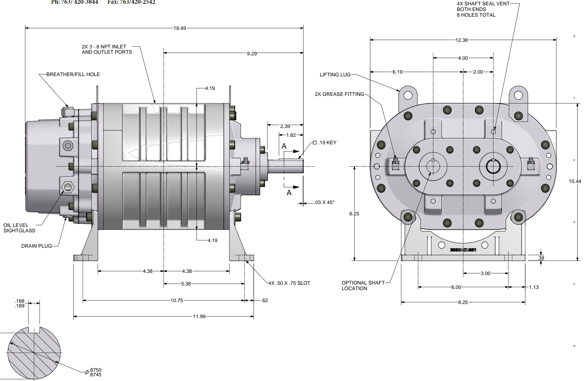
SECTION A-A SCALE 4 : 1
