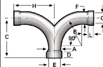
Standard Double 90° Y
